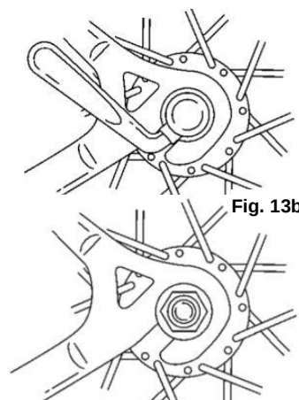
Ruota posteriore a bullone nei forcellini
